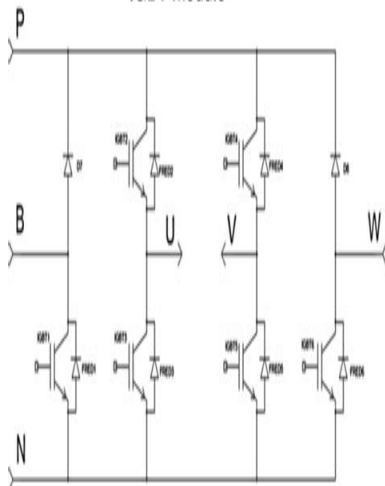
IGBT Module
